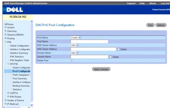
Abbildung 11-8. Poolkonfiguration - Anzeigen
