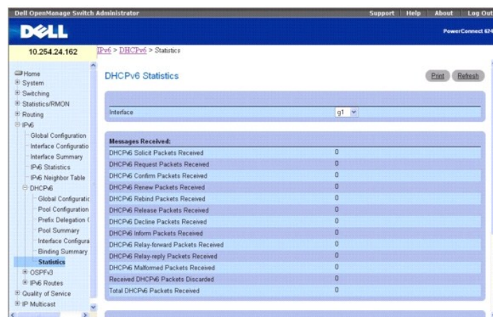
Abbildung 11-15. DHCPv6-Statistik
