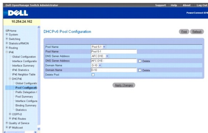
Abbildung 11-8. Poolkonfiguration - Anzeigen
