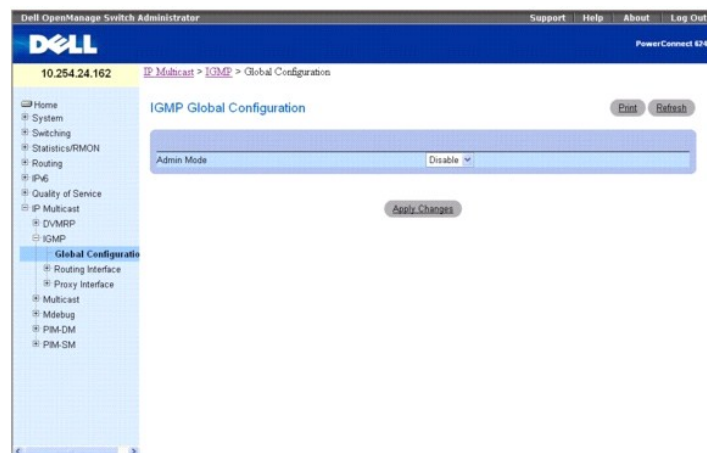
Abbildung 13-7. Globale IGMP-Konfiguration
